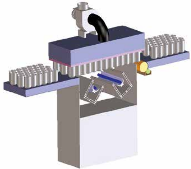
Layout einer typischen Rim Coating UV-Anlage
