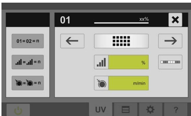
Bildschirmseite „Einstellungen – LED-Aggregat“
