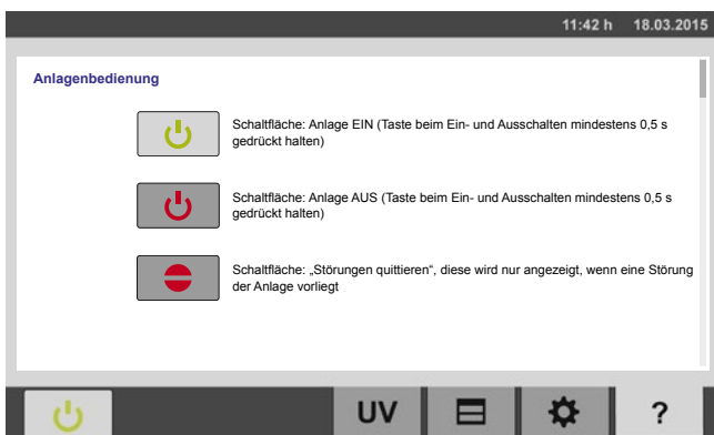
Bildschirmseite „Hilfe“
