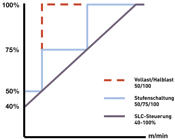
SLC Leistungssteuerung (optional ist auch eine elektronische Lampenregelung (ELC) erhältlich)
