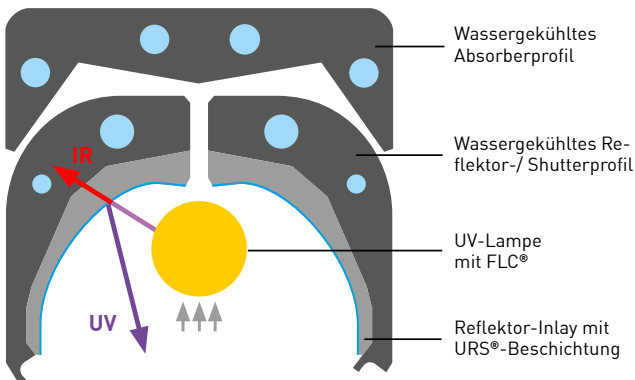
URS®-Reflektortechnologie
