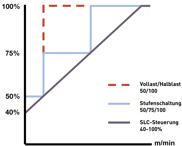
SLC Leistungssteuerung (optional ist auch eine elektronische Lampenregelung (ELC) erhältlich)
