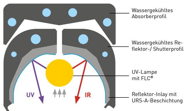
URS®-A-Reflektortechnologie
