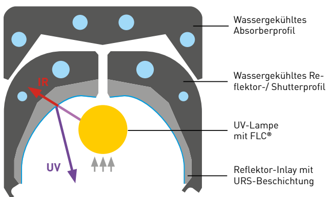
URS® -Reflektortechnologie
